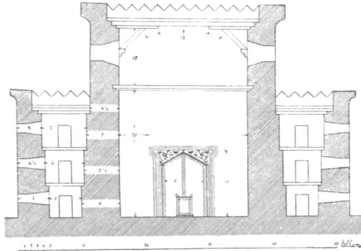
Doorsnede van het tempelhuis.
